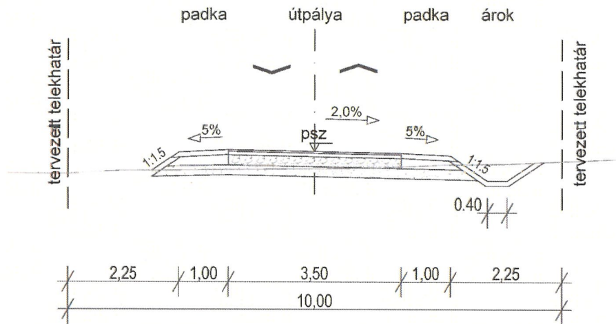
7. ábra Magánút javasolt mintakeresztmetszvény (M=1:100)
